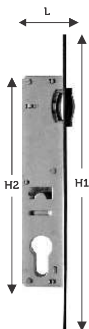
BL090 H1: 240 mm H2: 174 mm L: 37 mm
