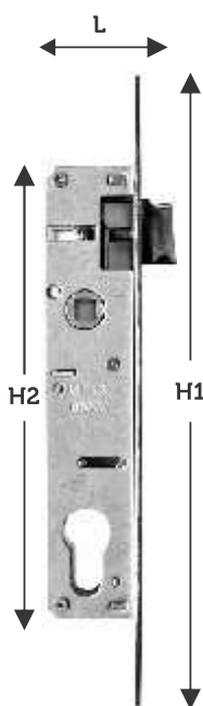
BL091 H1: 240 mm H2: 174 mm L: 37 mm
