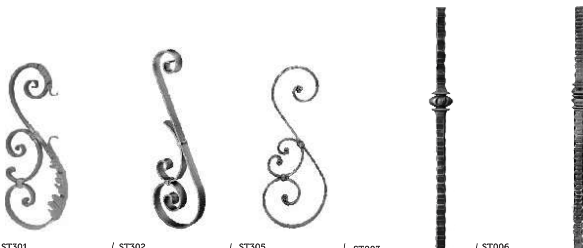
ST301 Sect: 30x8 mm H: 650 mm L: 300 mm
