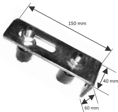
BL082 Ghidaj în forma de L cu 2 role de nylon Rolă: Ø 31 mm H 40 mm Grosime piesă metalică 5 mm
